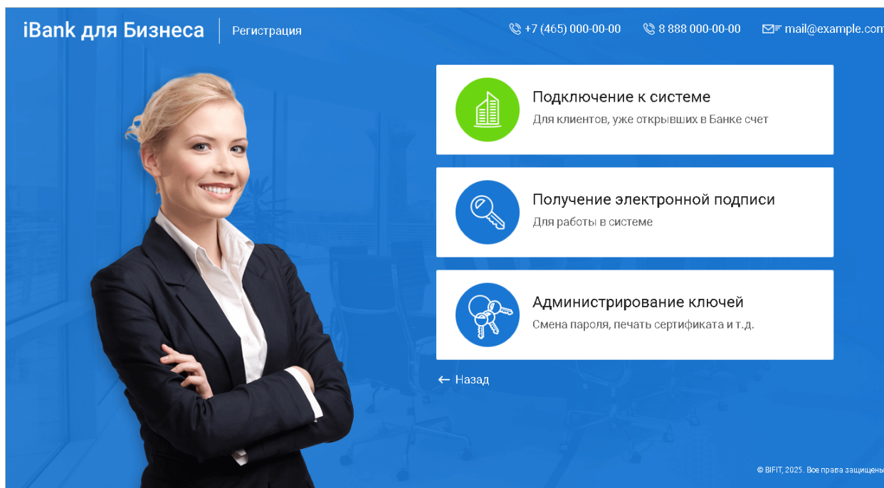
Рис. 5. Страница "Регистрация"
