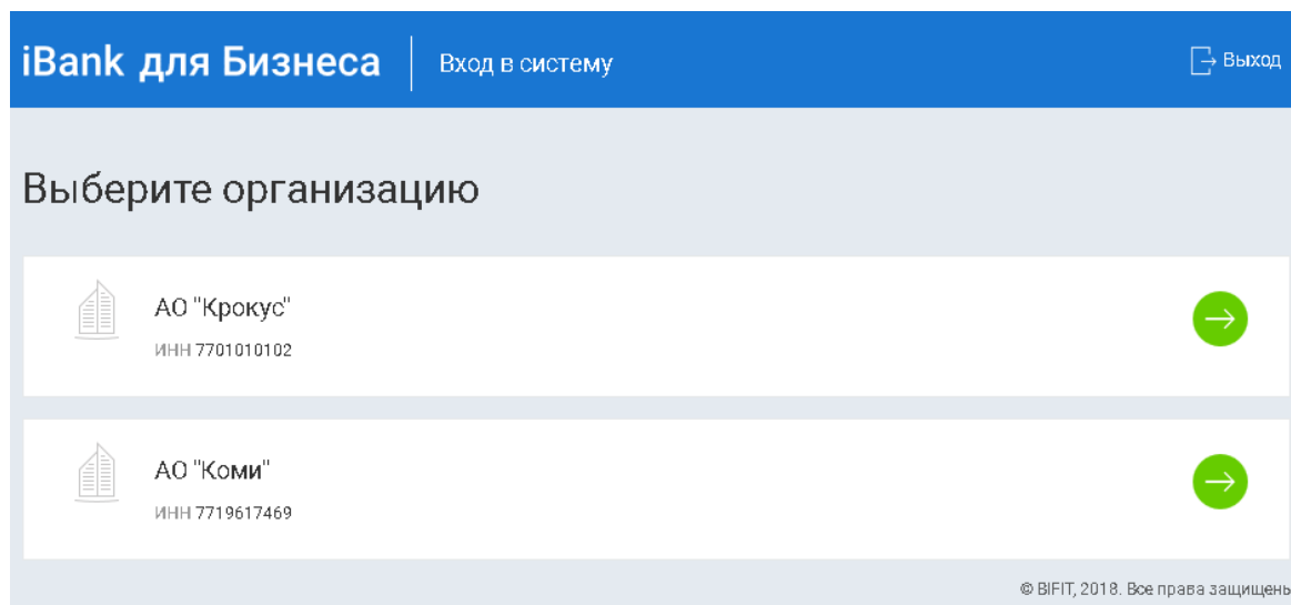
Рис. 41. Выбор организации
