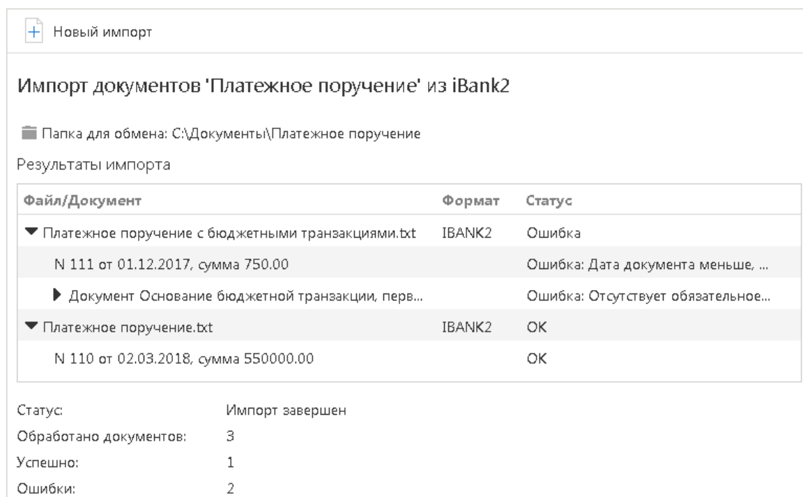
Рис. 484. Результаты импорта
