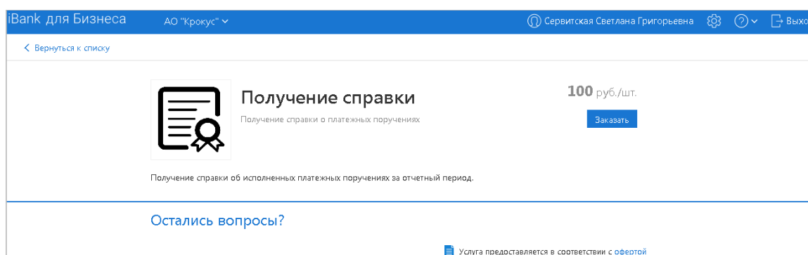
Рис. 142. Разовая услуга
