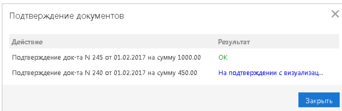
Рис. 461. Подтверждение документов
