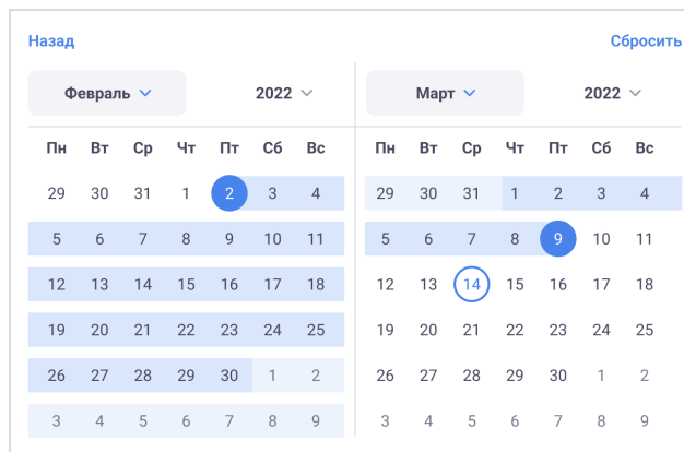
Рис. 21. Календарь
