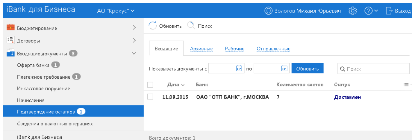
Рис. 397. Подтверждение остатков
