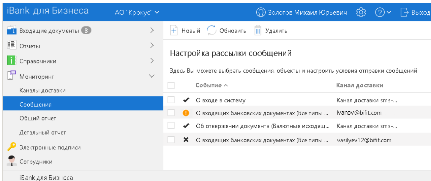
Рис. 439. Мониторинг. Сообщения
