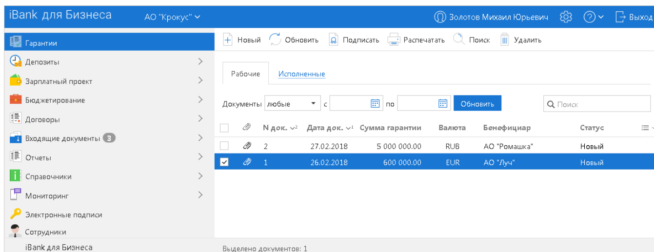
Рис. 325. Гарантии
