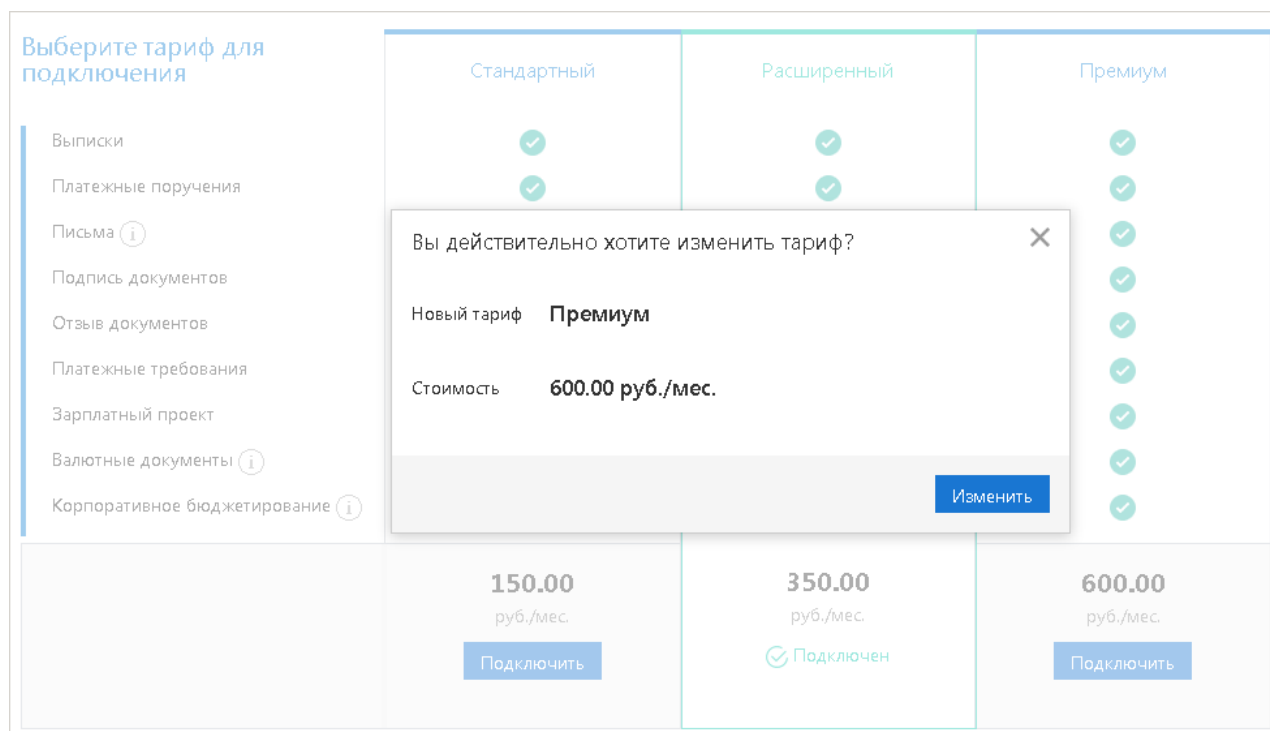
Рис. 139. Смена тарифа
