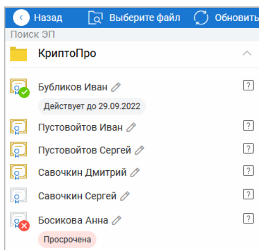
Рис. 11. Выбор ЭП
