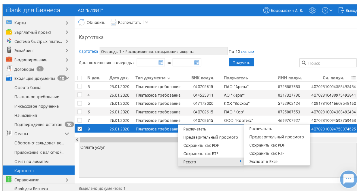
Рис. 405. Отчет «Картотека»
