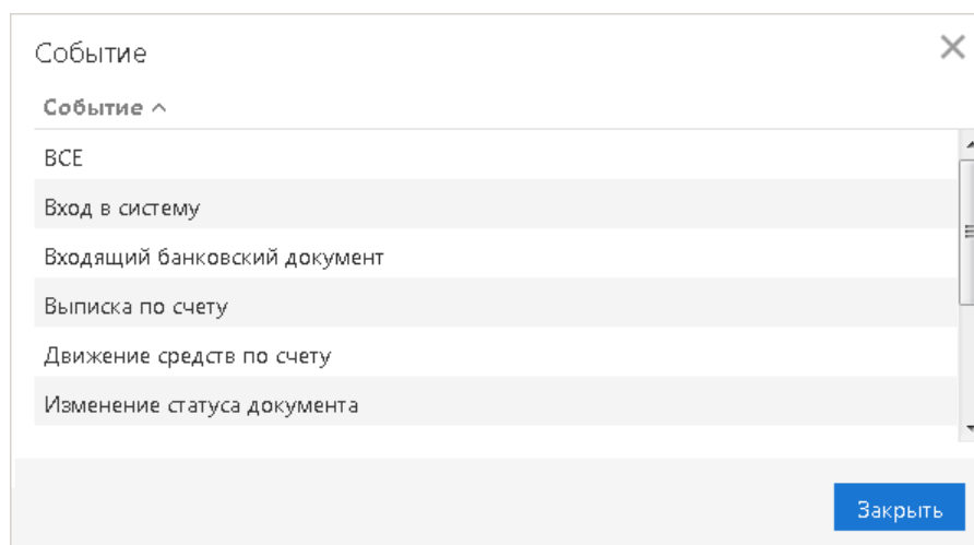
Рис. 446. Диалог "Событие"
