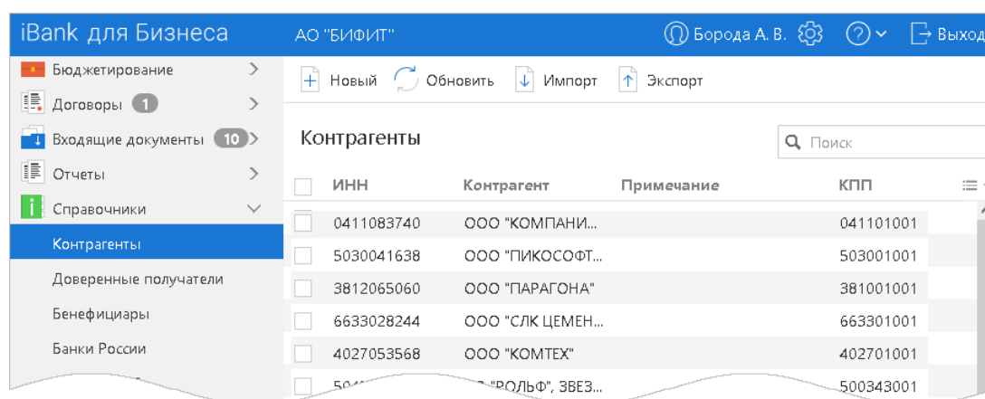
Рис. 416. Контрагенты
