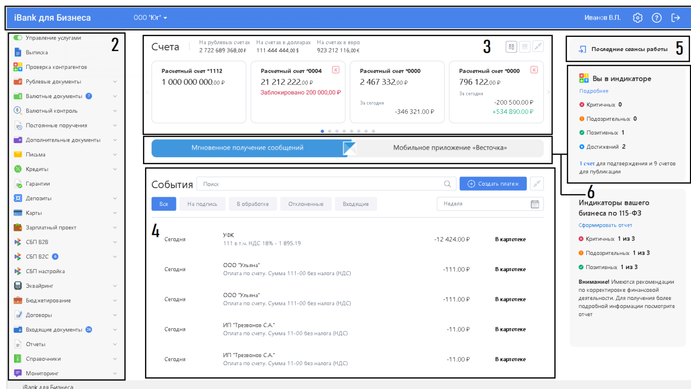
Рис. 15. Главная страница
