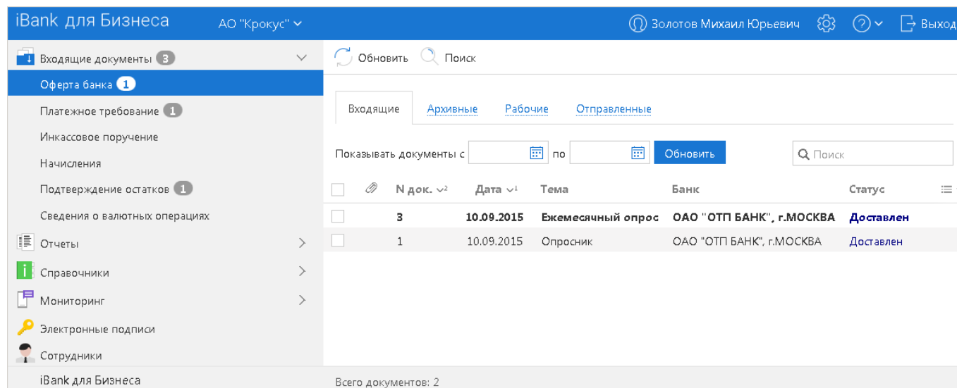
Рис. 386. Подтверждение сделки
