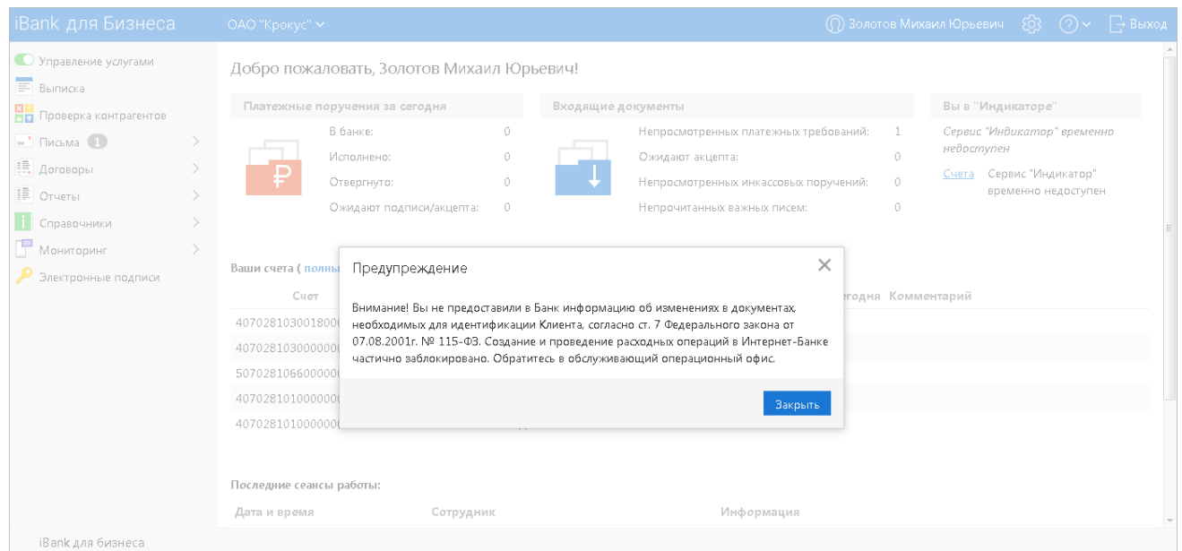
Рис. 30. Частичная блокировка
