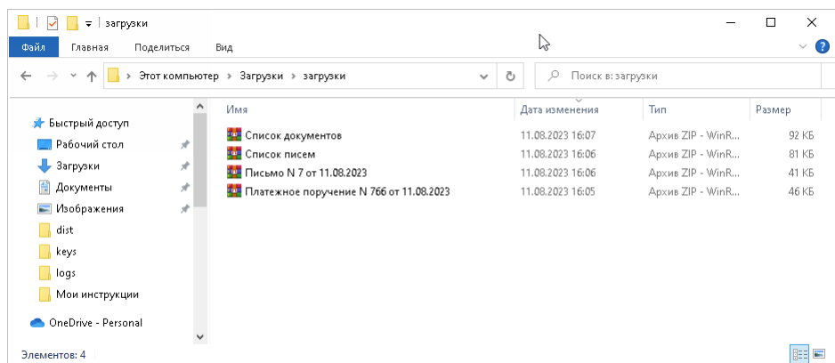
Рис. 99. Экспортированные документы
